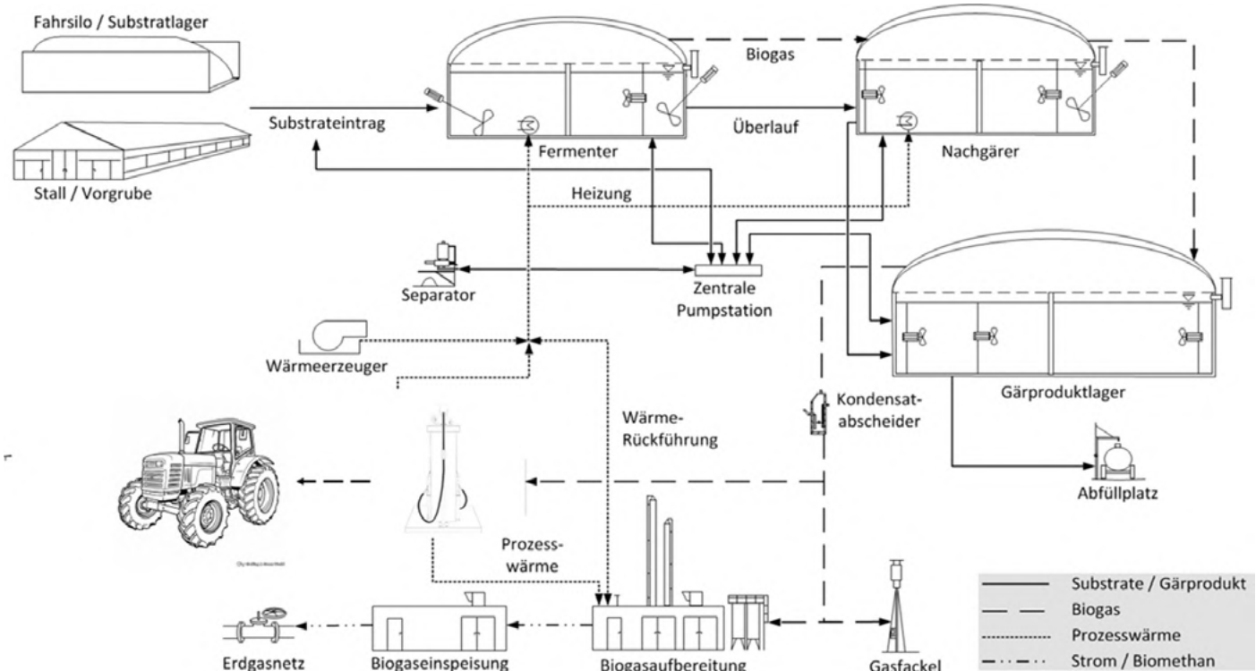
Figuur 13. Overzicht installatieonderdelen uit KTBL Probiogas-tool; de installatie bestaat uit een biogasinstallatie met een gecombineerde net-invoeding en CNG tankstation
